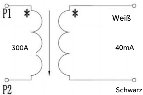
Elektrischer Schaltplan
